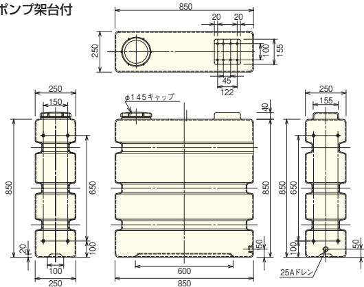
ポンプ攪拌機架台付
